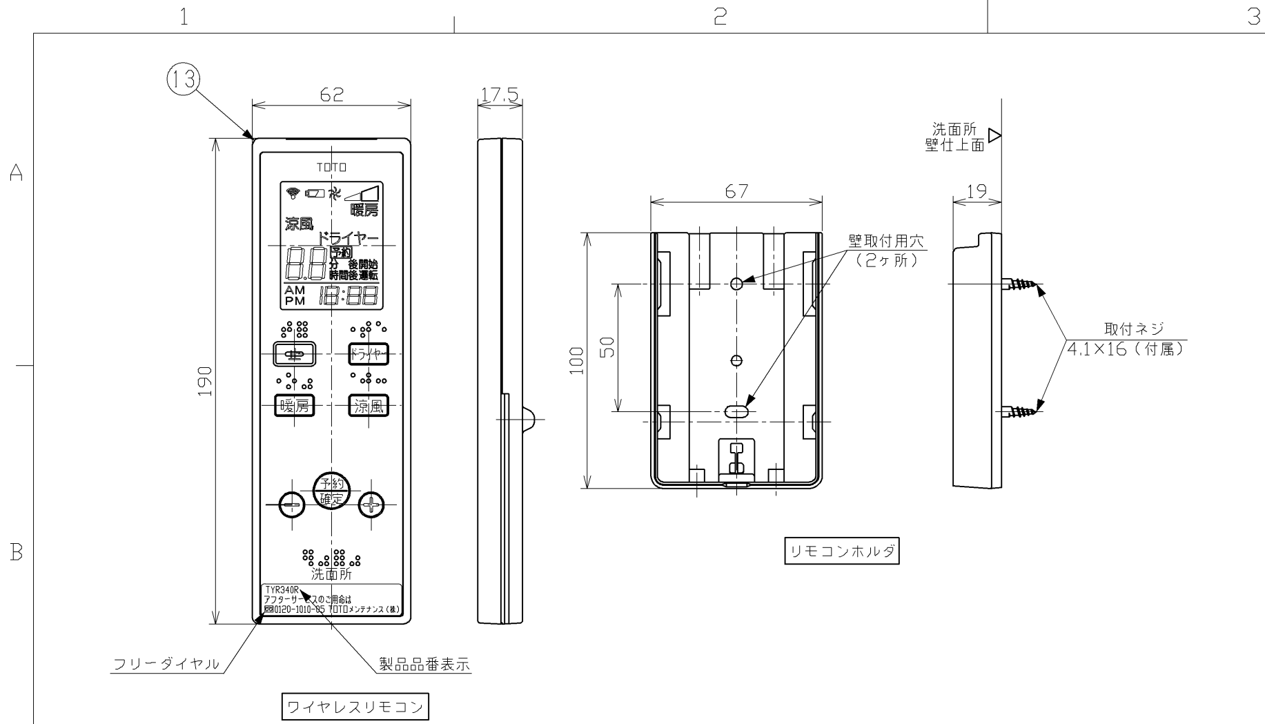
リモコン組品外観 (1:2)
