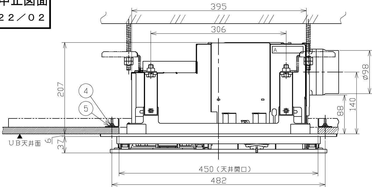
天井取付図
