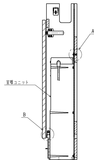
室暖ユニット固定詳細
