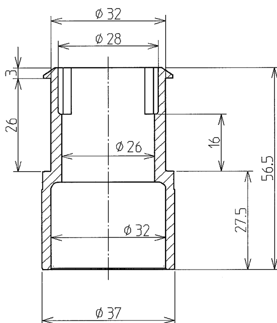
A-A断面
