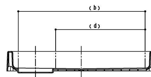
断面B-B
