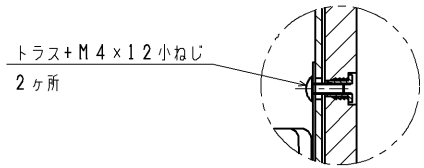
A部詳細 (S=1:2)
