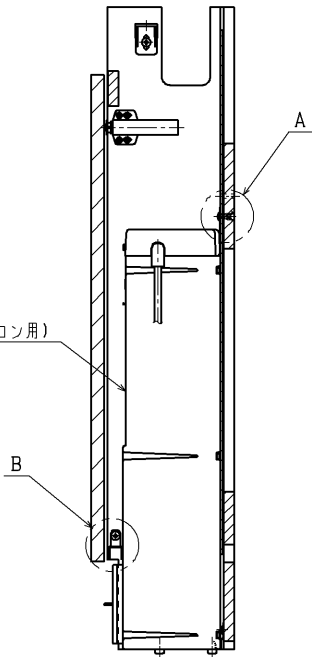
室暖ユニット固定詳細
