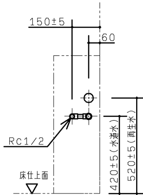
P 視図
