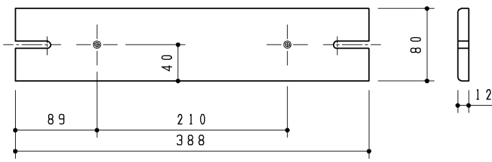
3 新築用木棧 (同梱部材)
