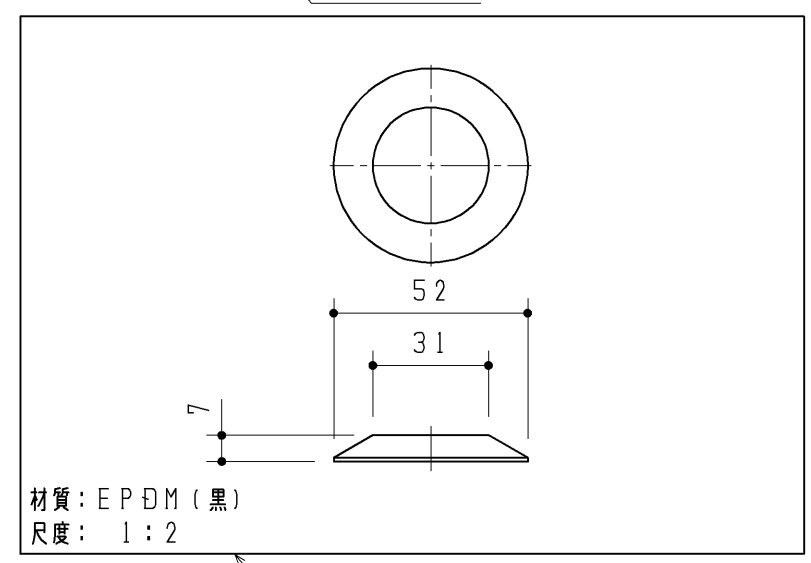
三角パッキン
