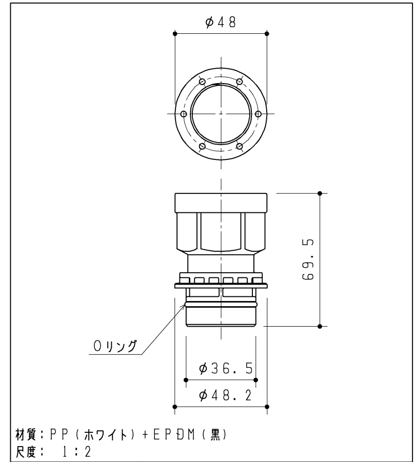
トラップ接続管
