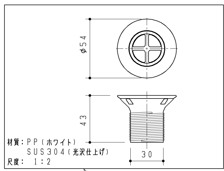
排水金具
