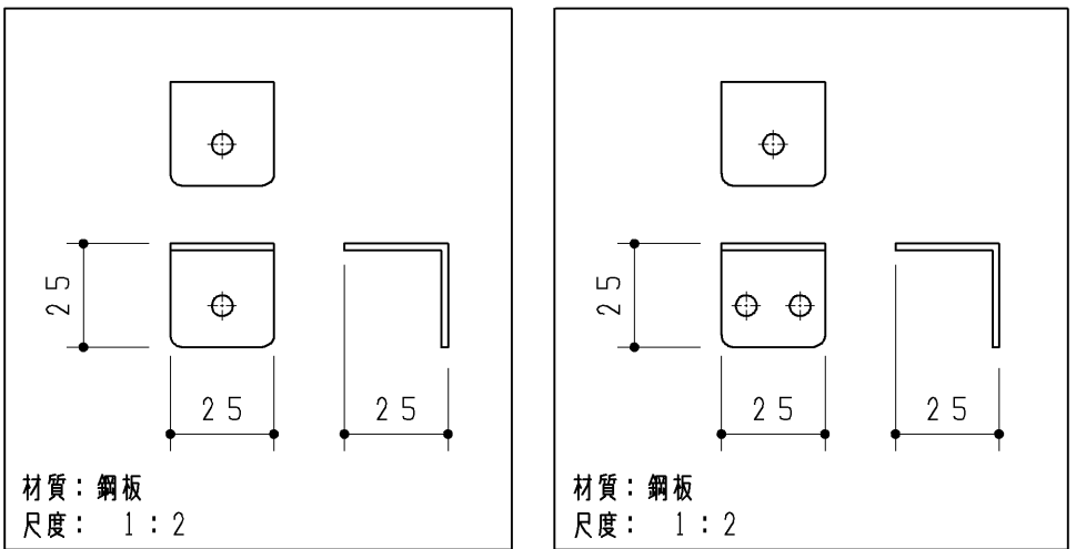
Lアングル
