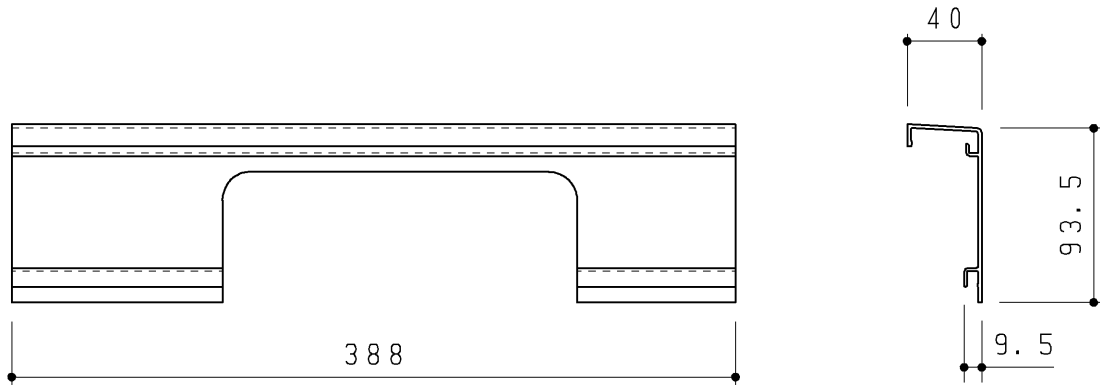
配管カバー-R（間口小）（ホワイト）
