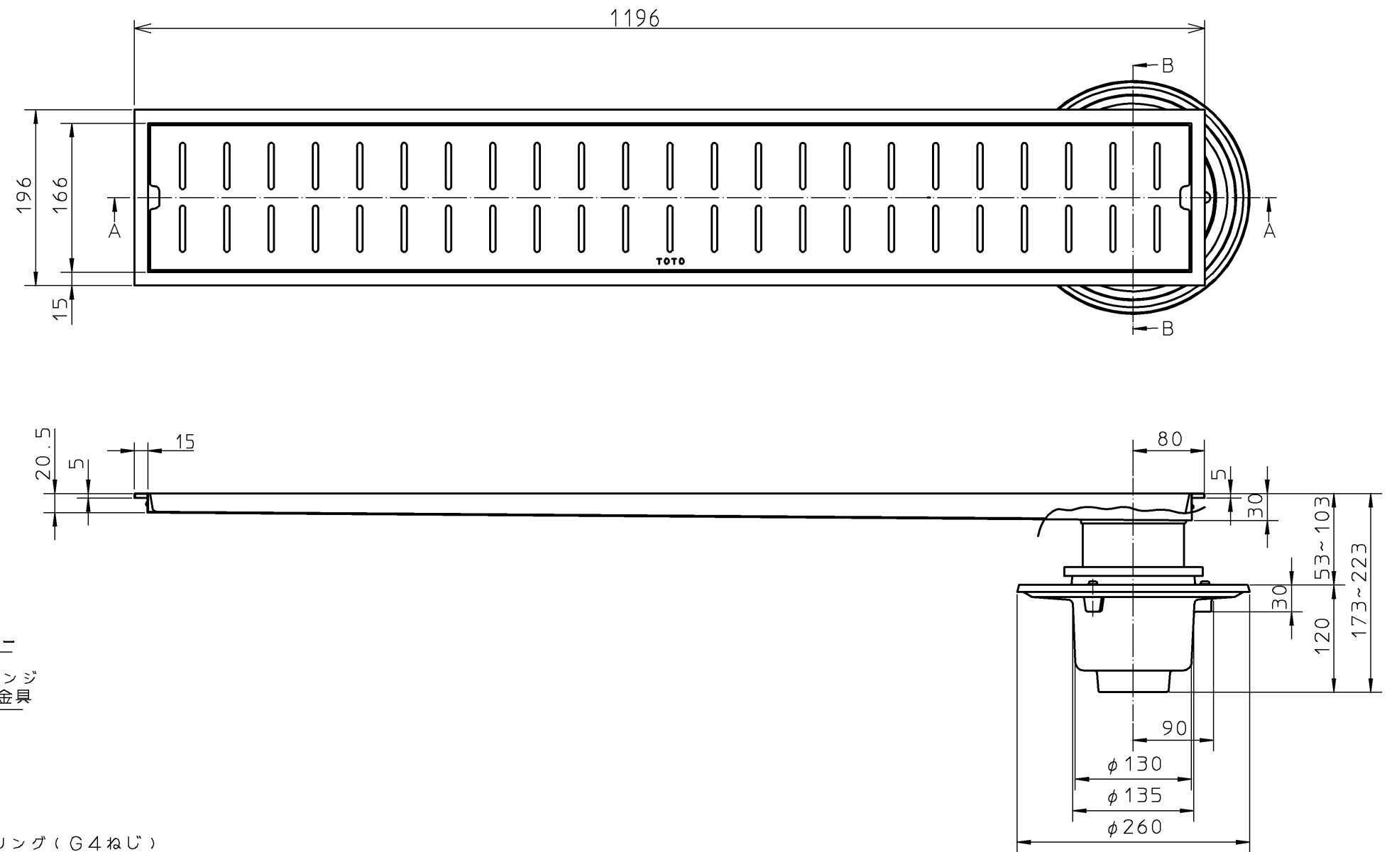
A-A 排水ユニット本体部断面
