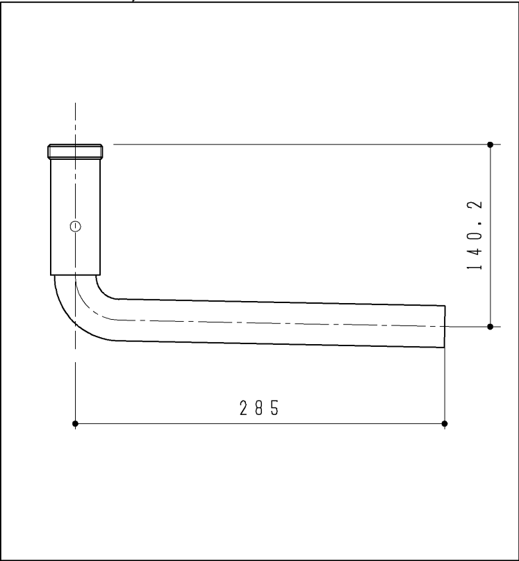
手洗排水管A(1200)
