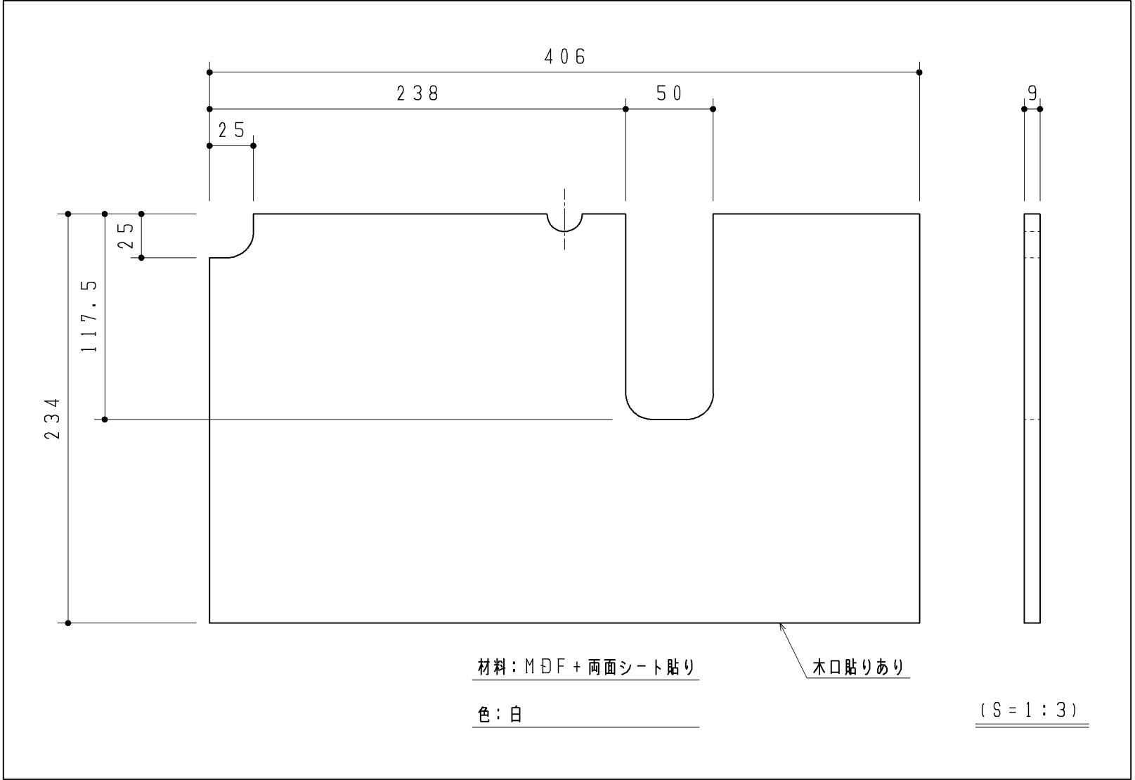
底板（1ヶ）
