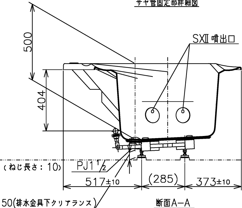
サヤ管固定部詳細図
