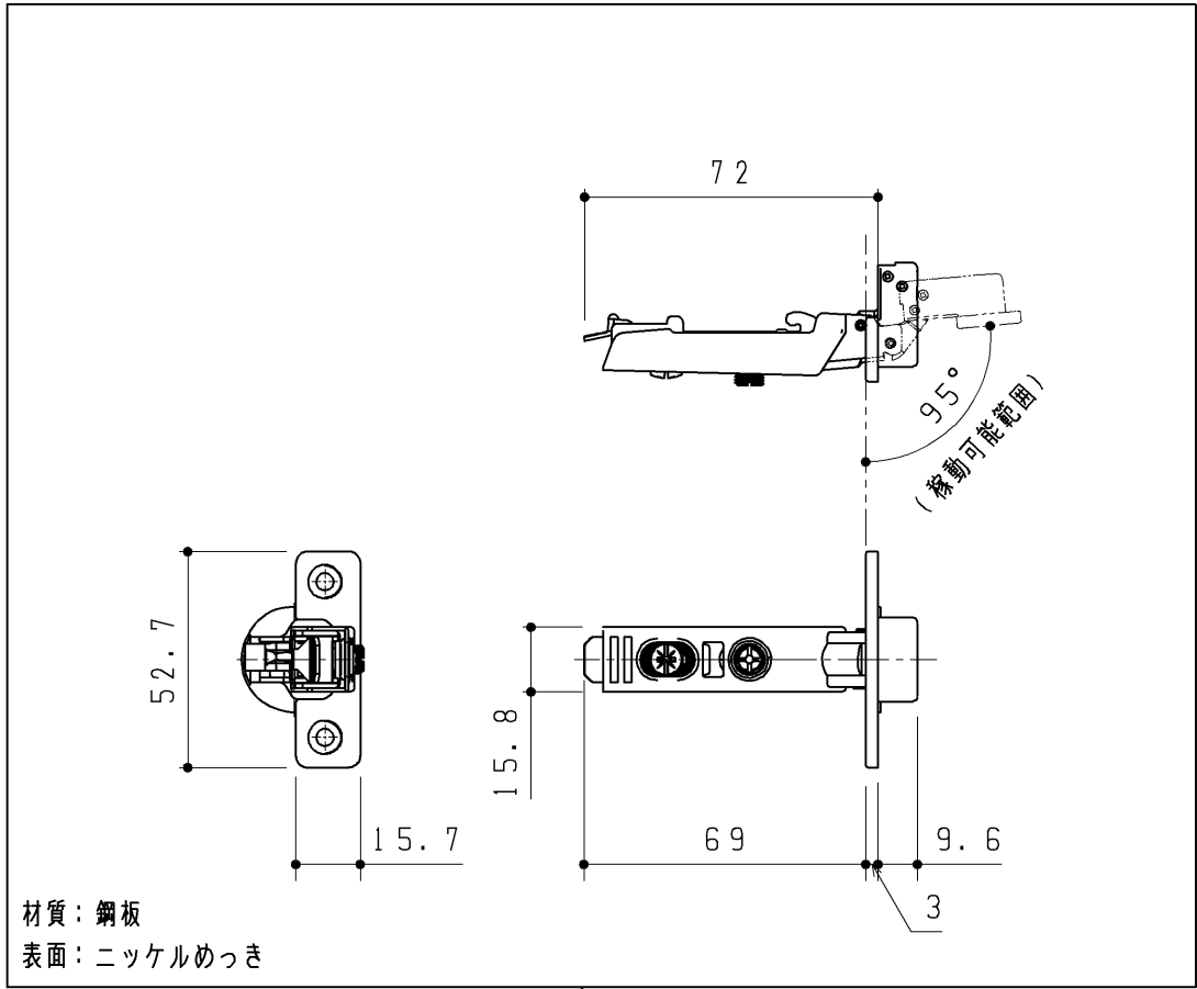
スライド丁番(2ヶ)
