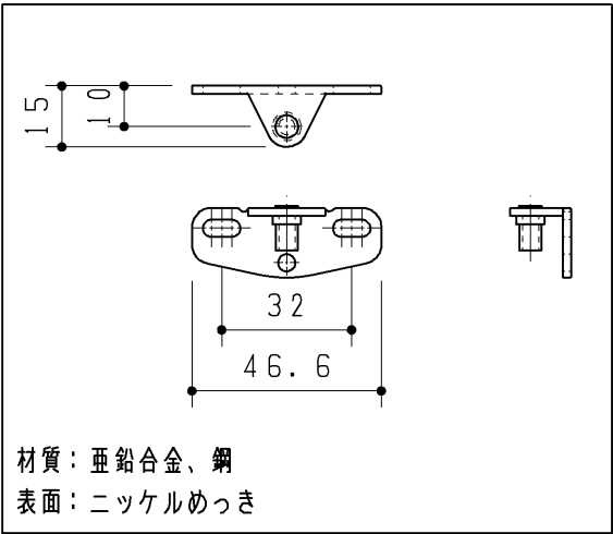
ダンパー取付用座金
