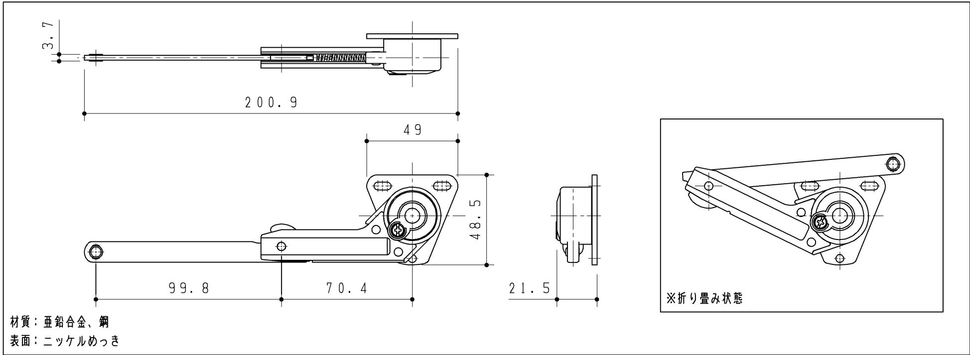
ダンパー本体
