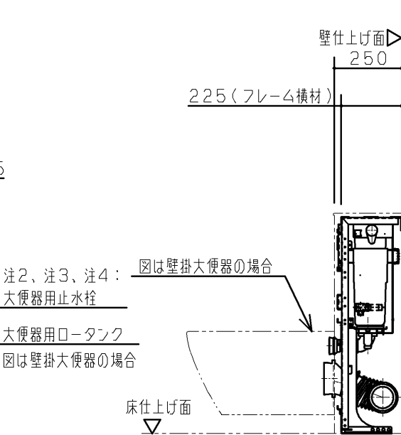
R 視図
