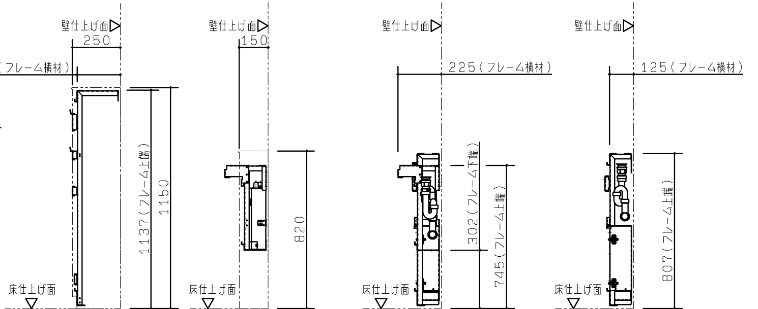
R 視図
