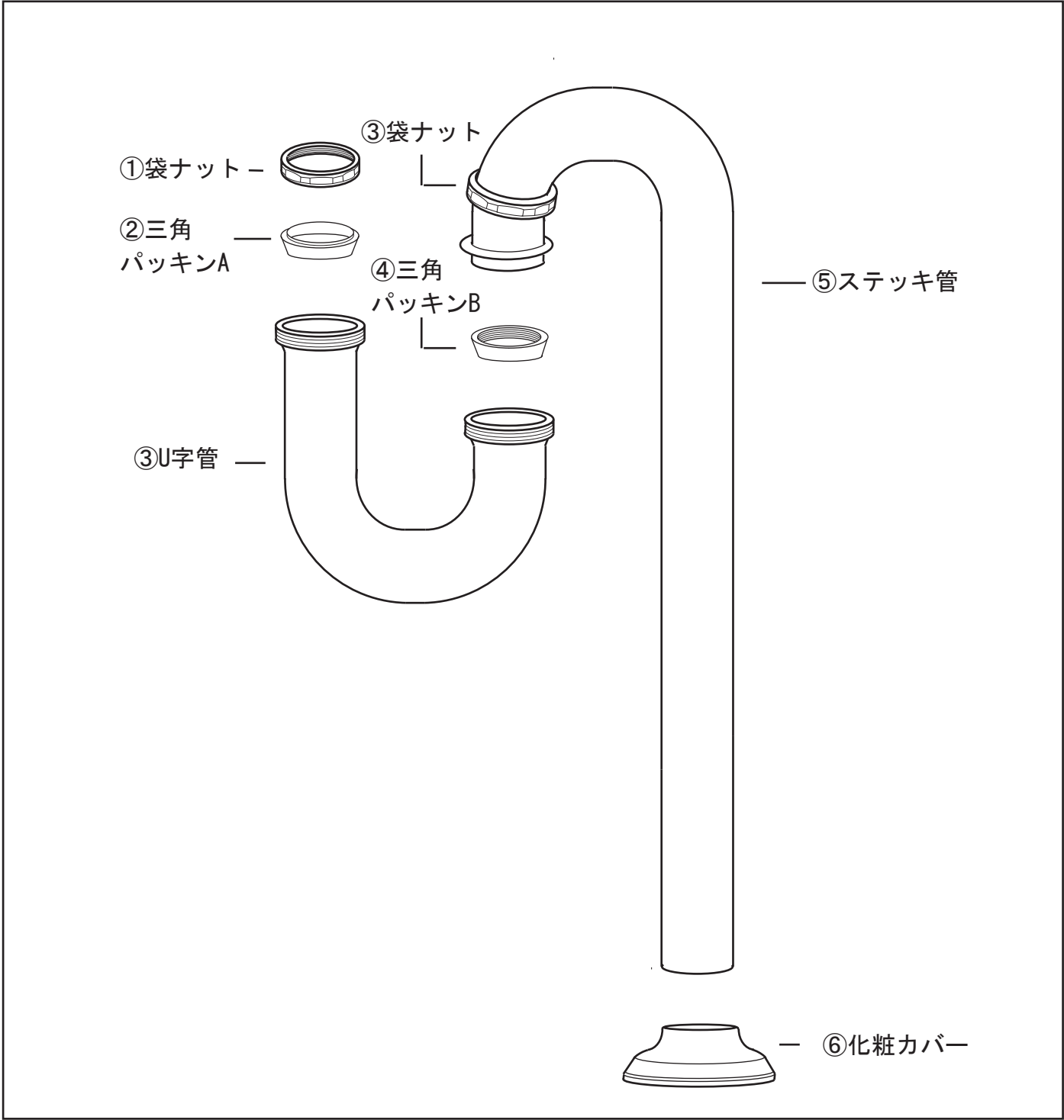
■ 製品図
