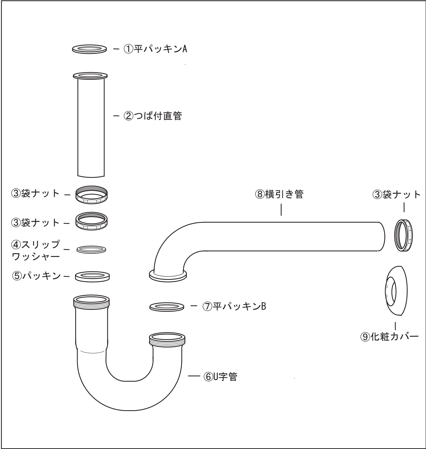
■ 製品図
