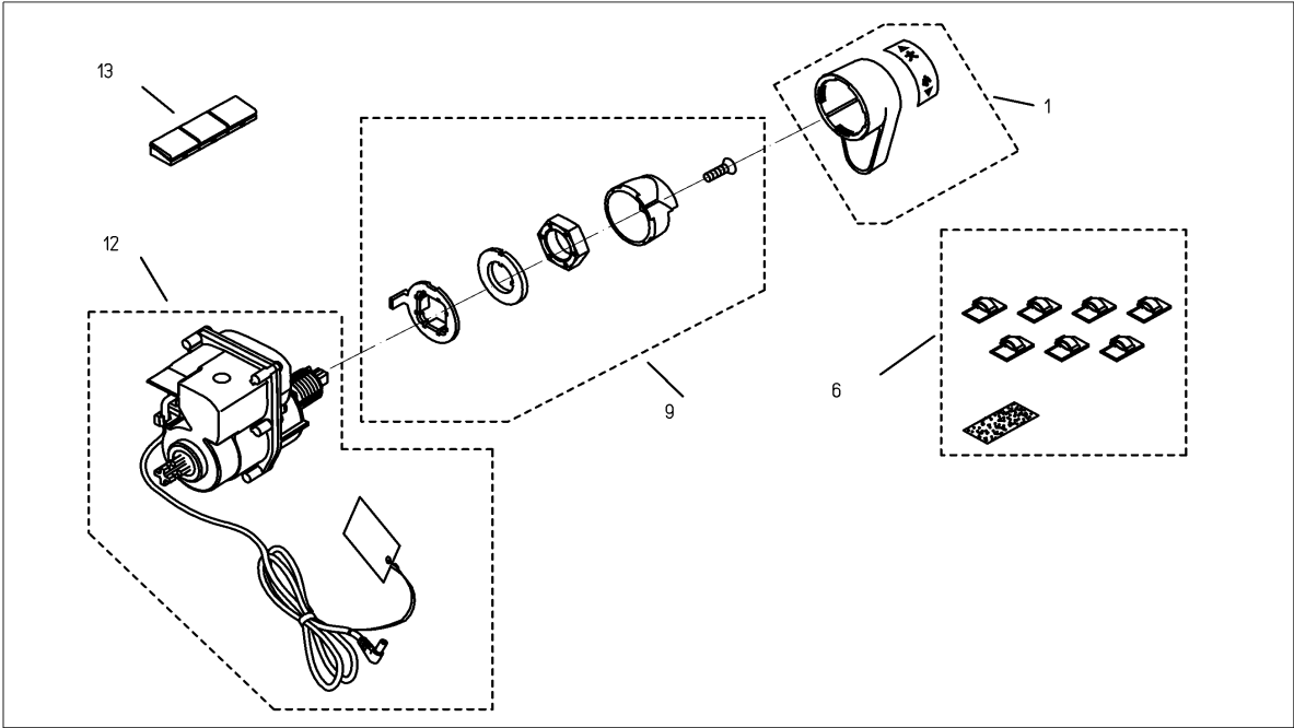
【分解図】
