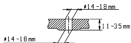
便器取付穴断面
