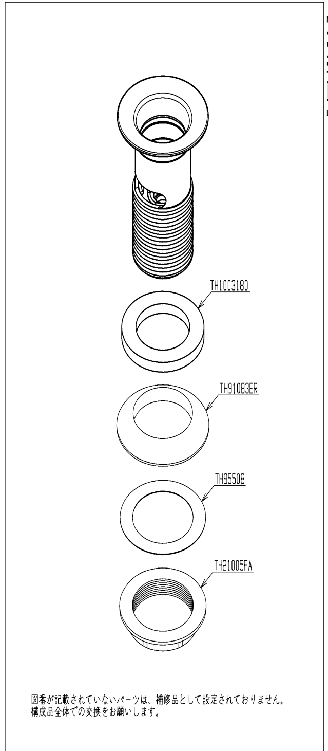
[ 分解図 ]
