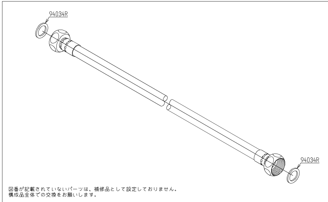
[外観図]
