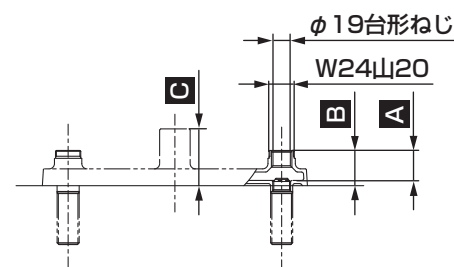
取付可能な水栓の主要寸法(mm)
