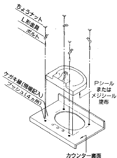
組立要領図
