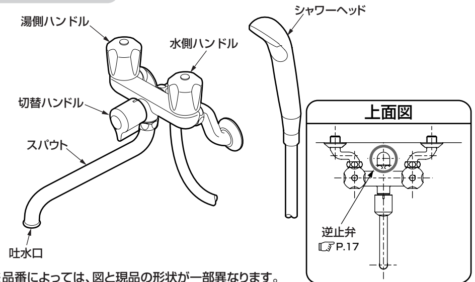
一時止水なしタイプ <TMS25型>
