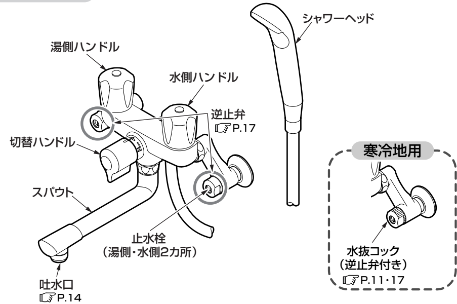
一時止水タイプ <TMG20型・TMJ20型・TMS20型>
