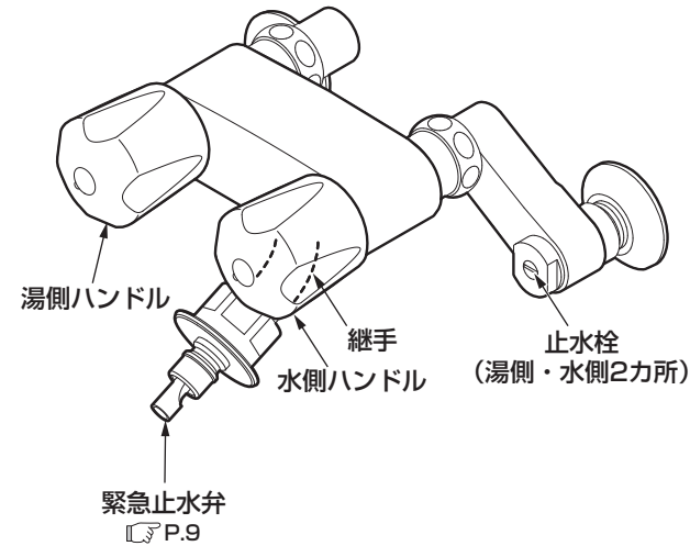
TW20型
