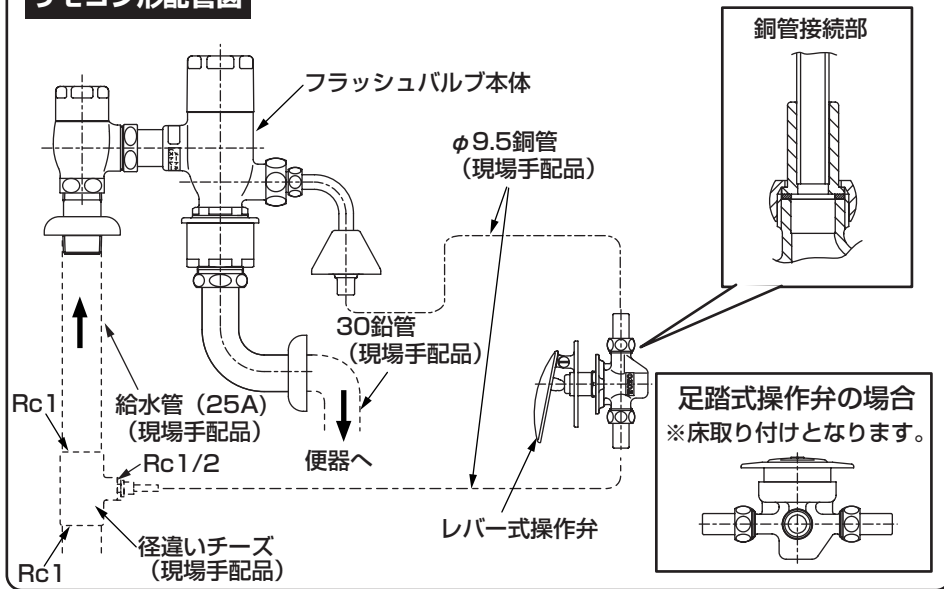
リモコン形配管図
