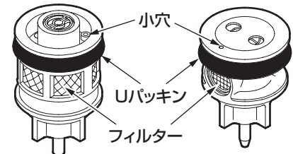
節水形フラッシュバルブ 普通形フラッシュバルブ
