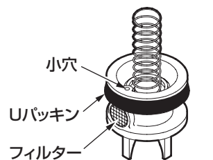
低圧形フラッシュバルブ
