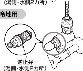
逆止弁 (湯側・水側2カ所)
