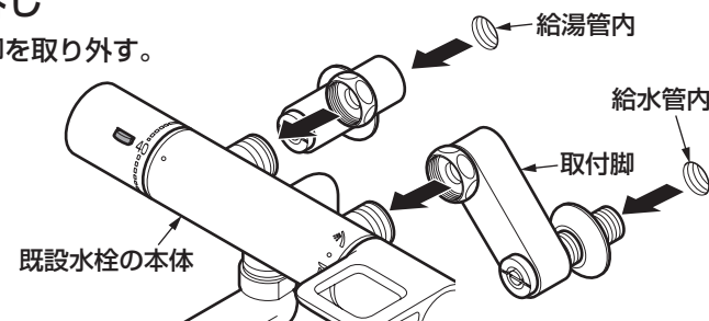
給湯管内
