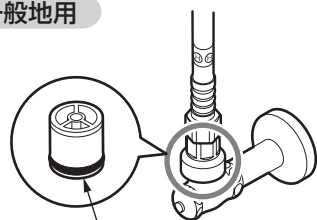
逆止弁 (湯側・水側2カ所)
