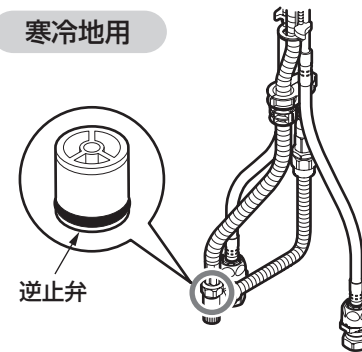
逆止弁 (湯側・水側2カ所)
