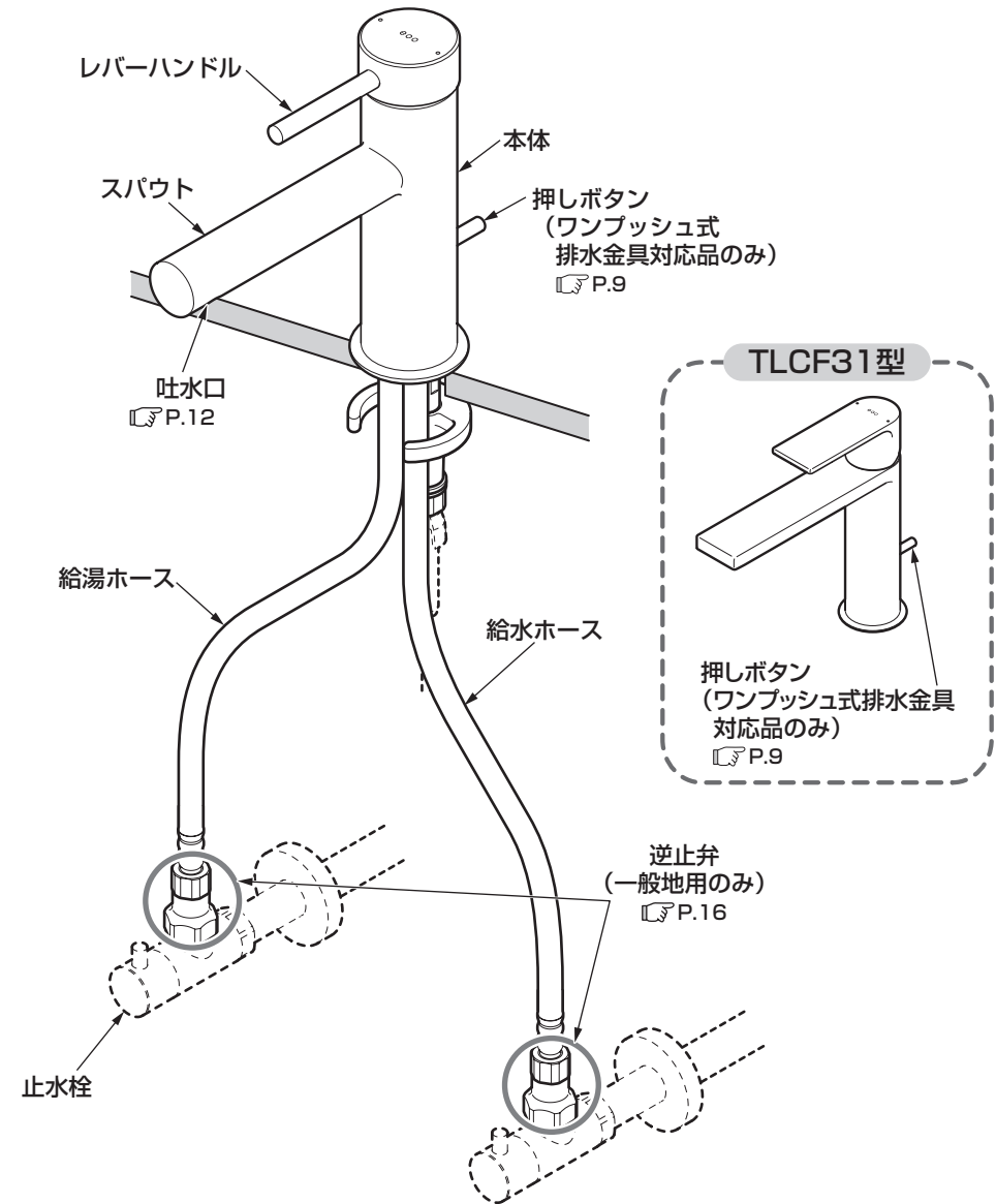
TLCC31型
