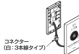
コネクター(白: 3本線タイプ)
