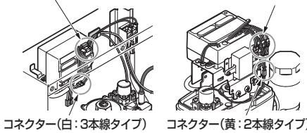
コネクター(白: 3本線タイプ)
