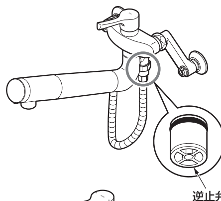
逆止弁 (湯側・水側2カ所)
