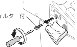
給水フィルター付 水抜栓
