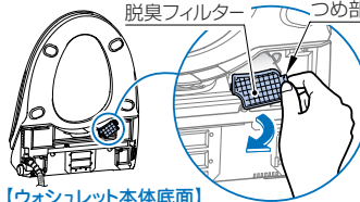
【ウォシュレット本体底面】
