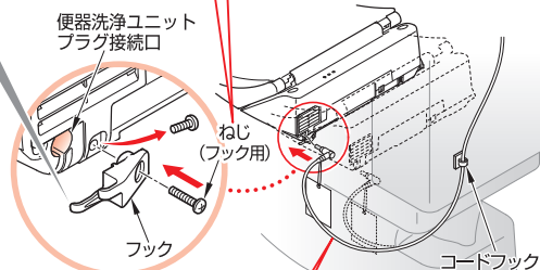
図はアプリコットF
