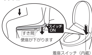
着座スイッチ (内蔵)
