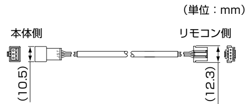
《リモコンコード詳細図》
