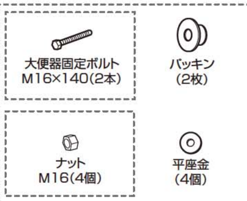
取付材 (1個)
