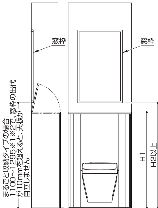
大便器後壁に窓がある場合
