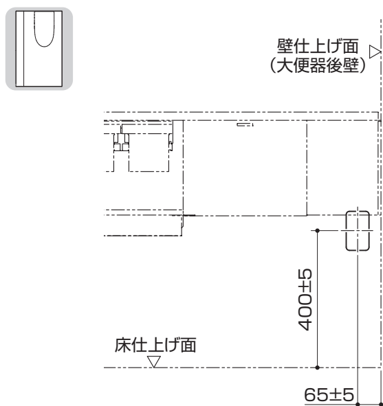
壁埋込式 1口コンセント
