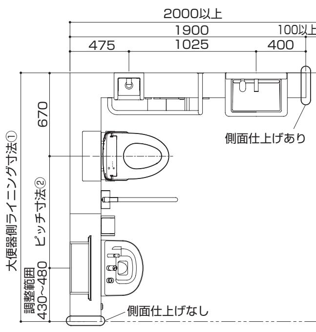
間口対応 (2000mm ~ 2400mm)
