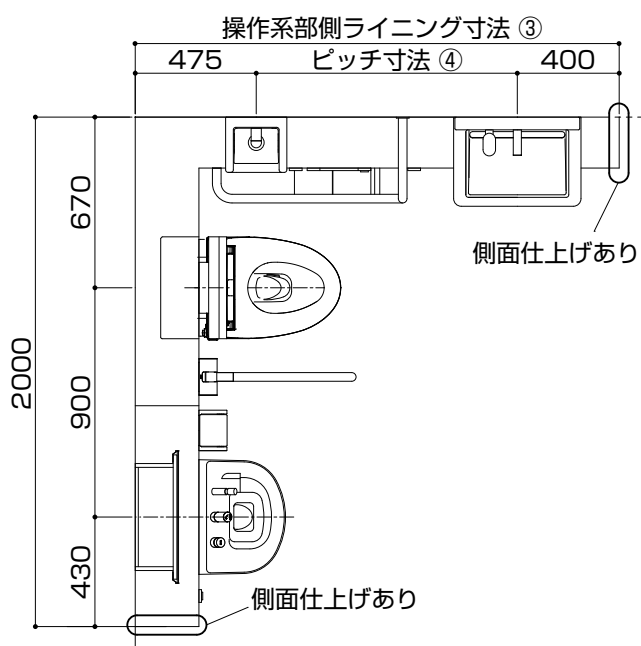
間口固定 (2000mm)
