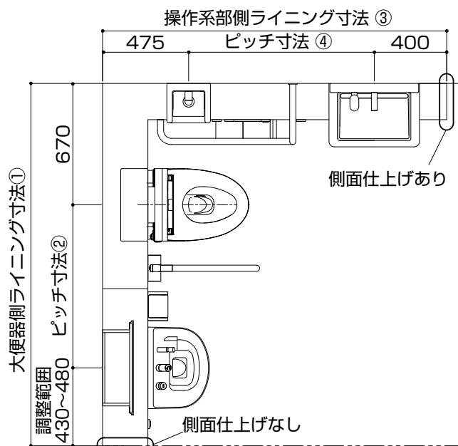
間口対応 (2000mm~2400mm)
