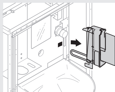
③回転させて引き抜く
