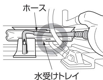
【正しいホースの位置】
