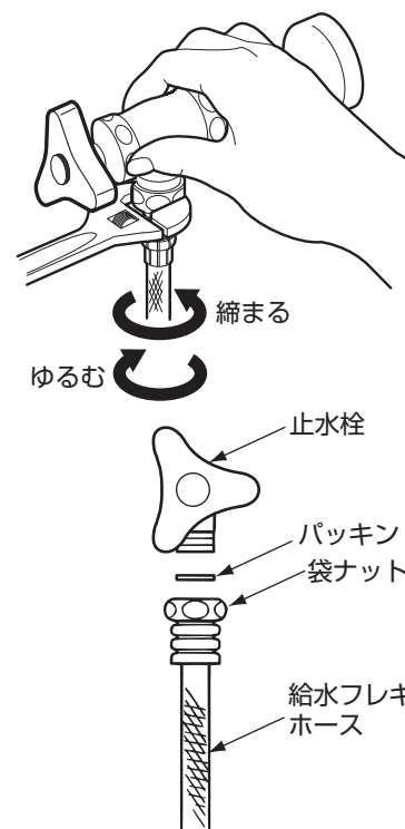
モンキーレンチ
