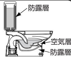
<参考>防露便器、タンクの構造
