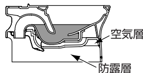
<参考>防露便器
